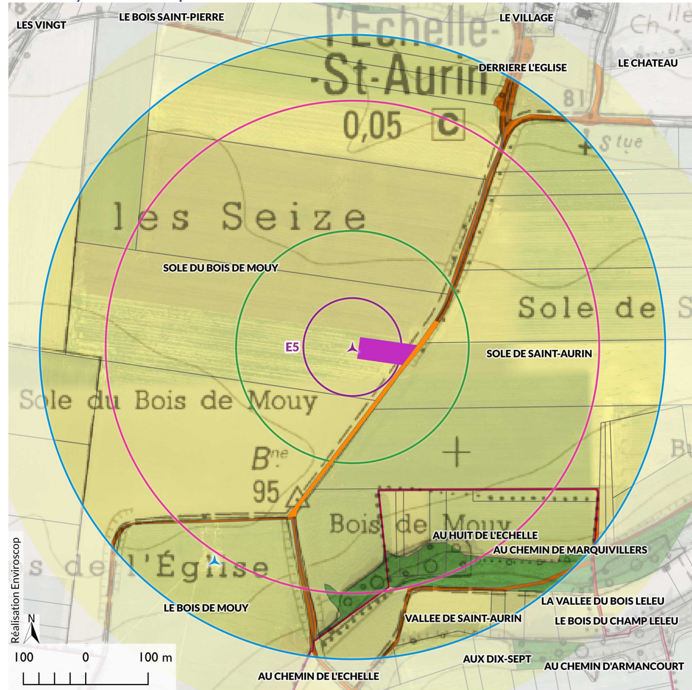
Carte 8 : Synthèse des risques de l'éolienne E5
