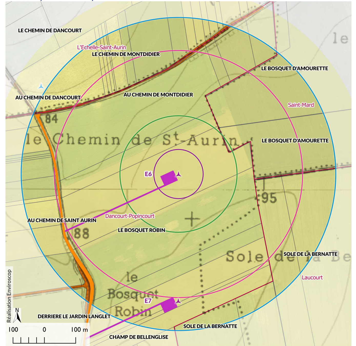
Carte 9 : Synthèse des risques de l'éolienne E6
