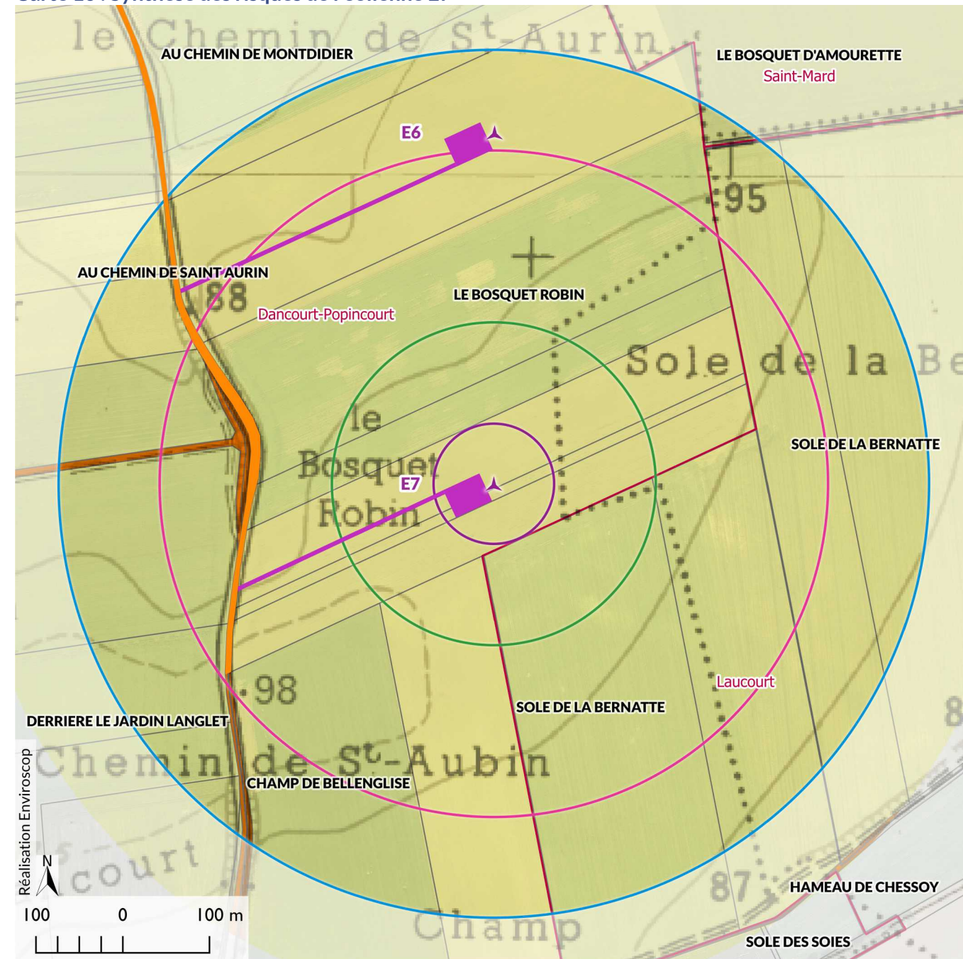
Carte 10 : Synthèse des risques de l'éolienne E7
