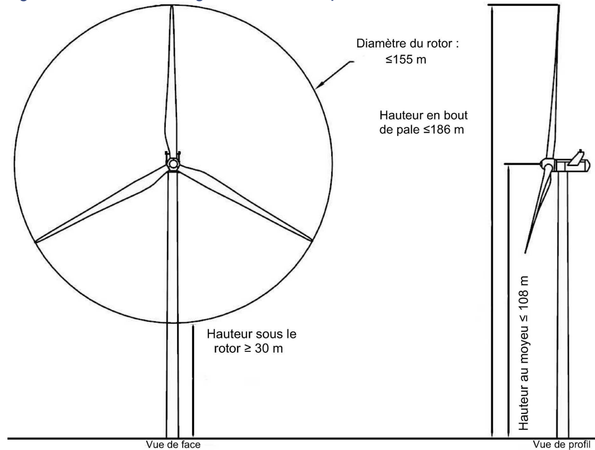
Figure 3 : Vue d'ensemble du gabarit de l'éolienne pour l'éolienne E7
