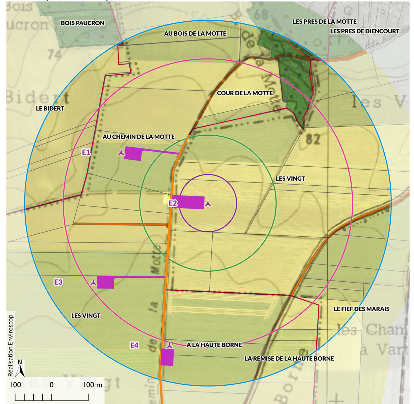
Carte 5 : Synthèse des risques de l'éolienne E2
