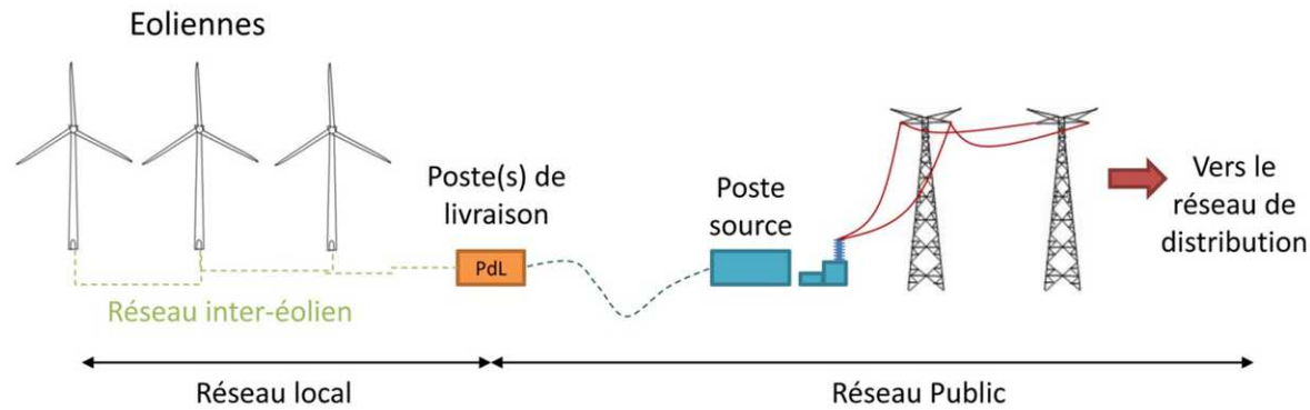
Figure 1 : Principe du raccordement électrique des installations
