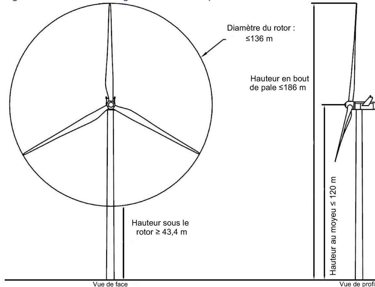
Figure 3 : Vue d'ensemble du gabarit de l'éolienne pour l'éolienne E7
